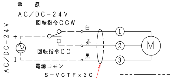
ロータリーアクチュエーター結線図
