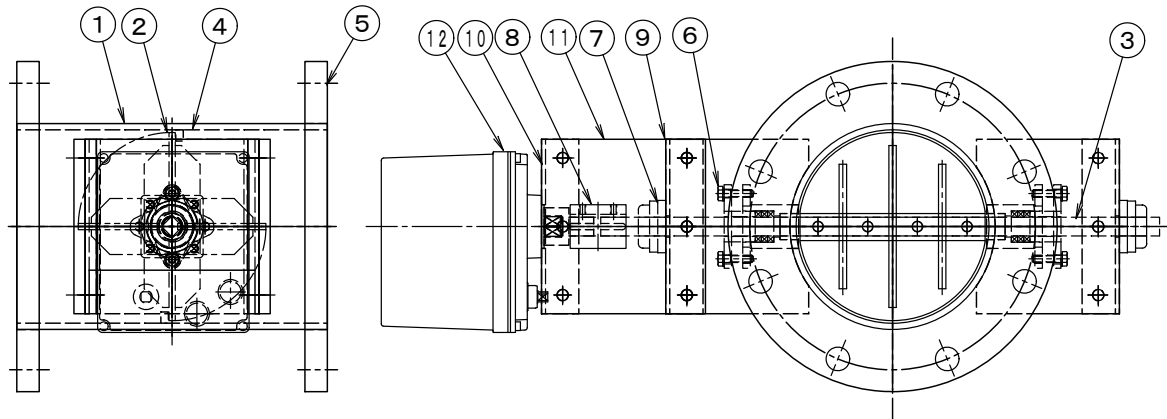
外形図
