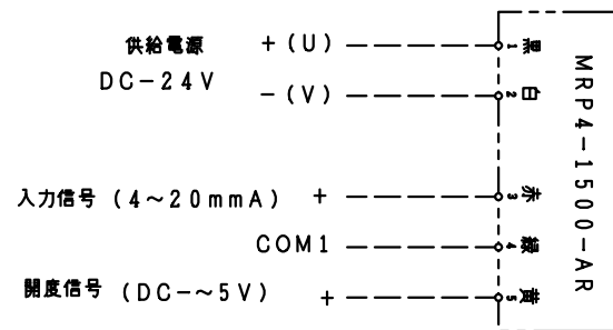
電気結線図
